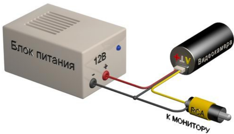
Схема подключения видеокамеры VB193CH-P37C
