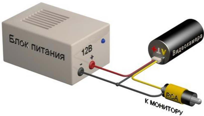
Схема подключения видеокамеры VB21HQX-R36
