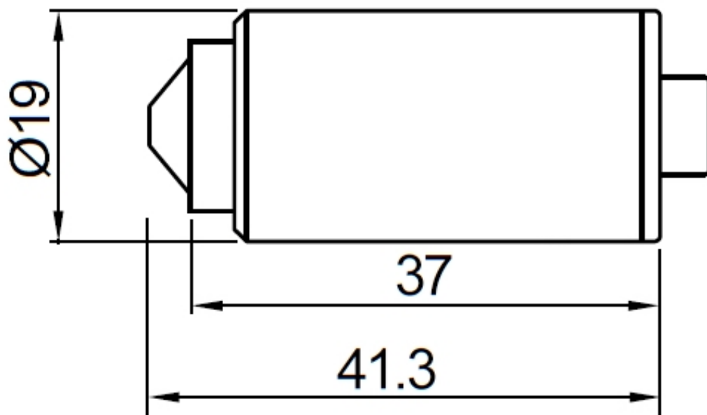
Размеры камеры видеонаблюдения VCL-P422H-P4
